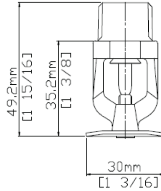
PENDENT SPRINKLER
